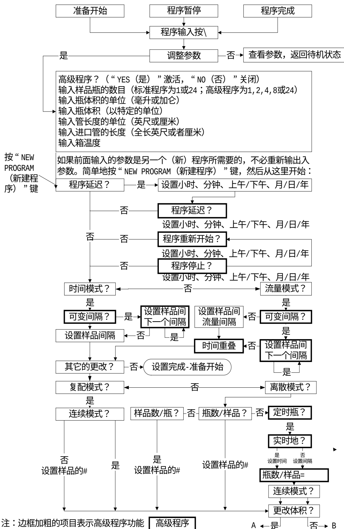
程序流程图
